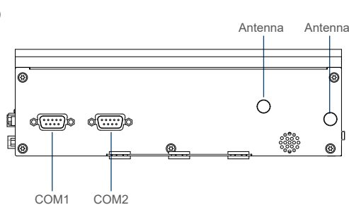
Right I/O
